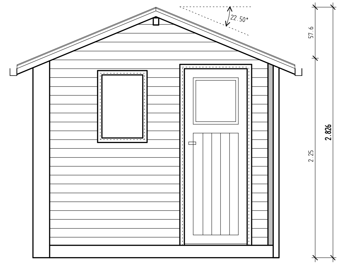
Vorderansicht
