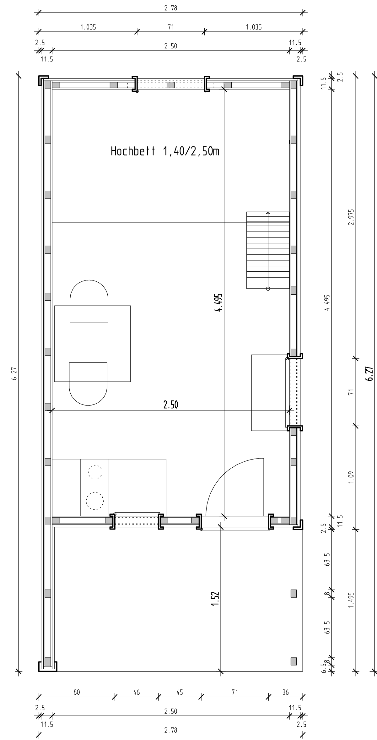
Grundriss
